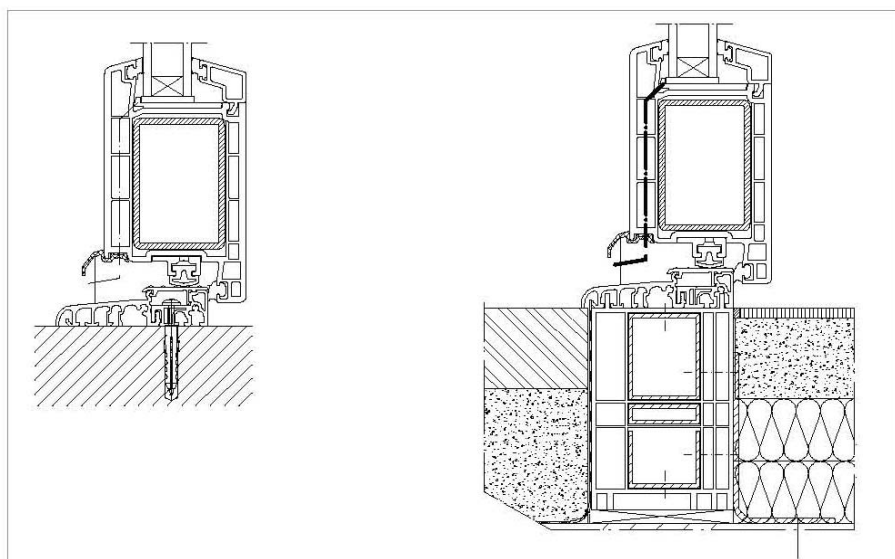
Rys. 20. Mocowanie progu
