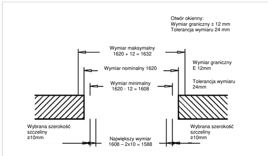
Rys. 4 Pasowanie - rama okienna
